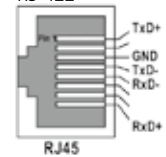
RS-422
